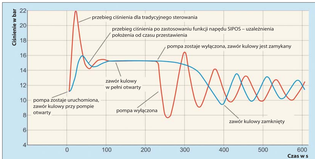
Ilustracja 5. Typowy przebieg ciśnienia zmierzony w pompie lub za armaturą pompy (zawór kulowy) rejestrowany podczas rozruchu lub wyłączania stacji pomp. Niebieska krzywa wyraźnie pokazuje tłumienie uderzeń ciśnienia po zastosowaniu funkcji napędu SIPOS 5 – uzależnienia położenia od czasu przestawienia
