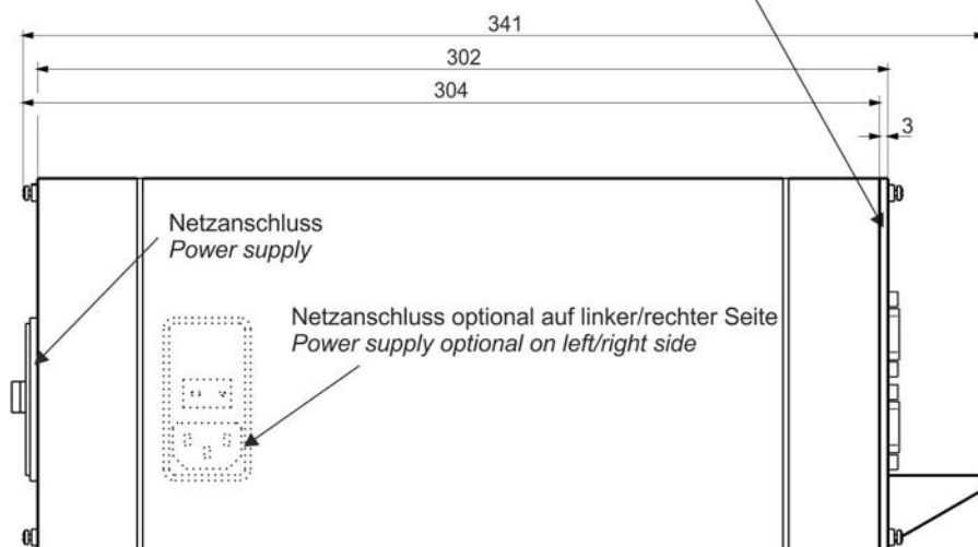
Seitenansicht Side view
